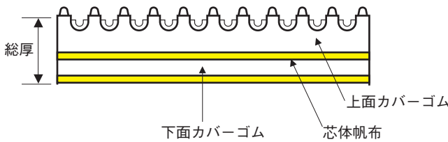
ベルト断面構造図
